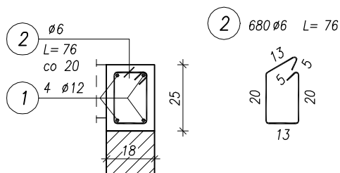
W-1 wieniec skala 1:20
